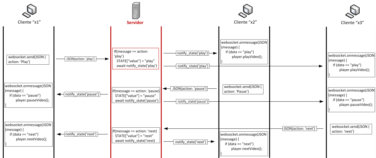
Figura 20 – Protocolo da funcionalidade Play, Pause e Next com 3 clientes conectados
