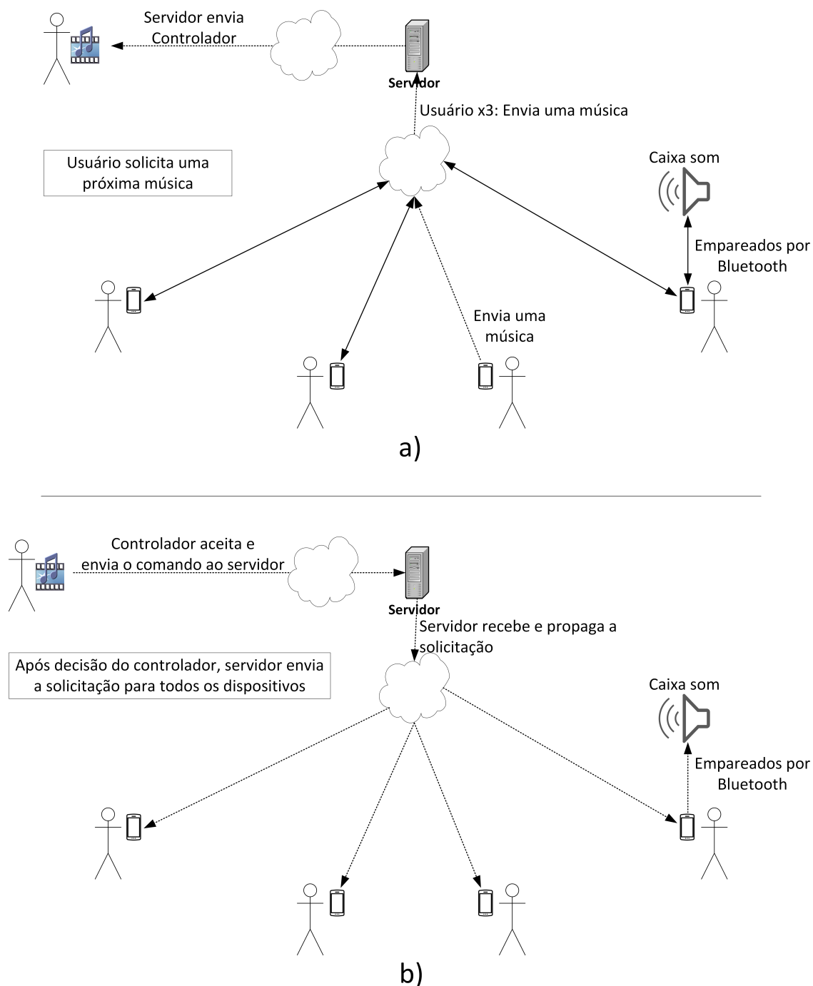
Figura 17 – Cenário 3 - Troca de mensagens
