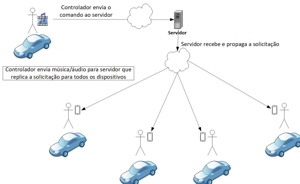
Figura 18 – Cenário 4 - com veículos
